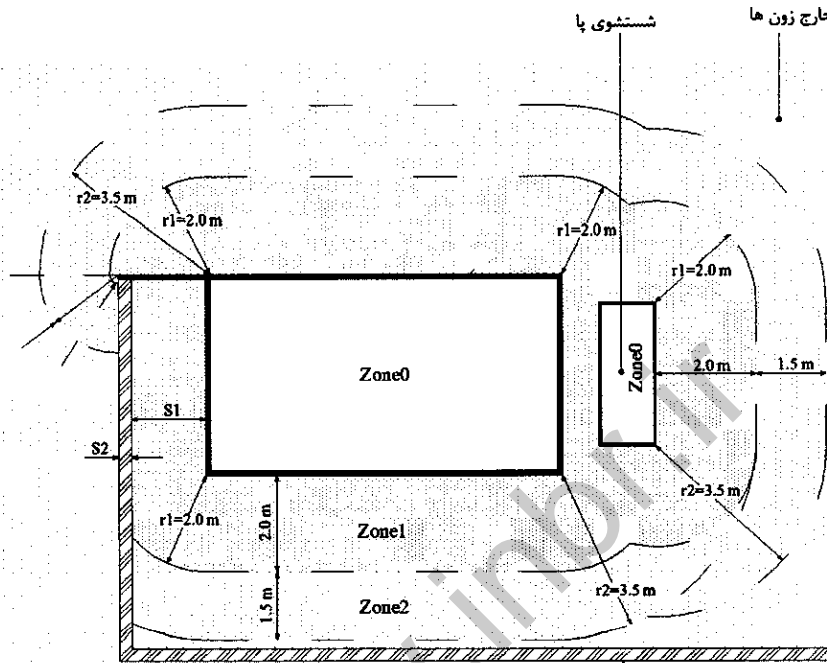
دیوار جداکننده ثابت = S1 = فاصله استخر از دیوار جداکننده ثابت ضخامت دیوار جداکننده ثابت = S2
