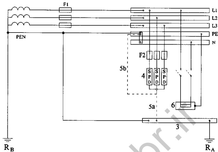
شکل ۱۳-۱-۳-۱۶-۴:۱ طرحواره نصب برقگیر حفاظتی در شبکه توزیع سیستم نیروی TN (سه فاز)
