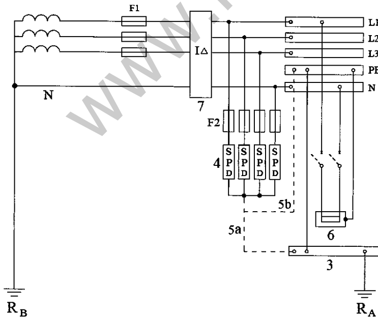
شکل ۱۳-۱-۳-۱۶-۴:۲ طرحواره نصب برقگیر حفاظتی در شبکه توزیع سیستم نیروی TT با قرارگیری برقگیر حفاظتی در طرف تغذیه بار و بعد از کلید حفاظتی جریان باقی مانده (RCD)
