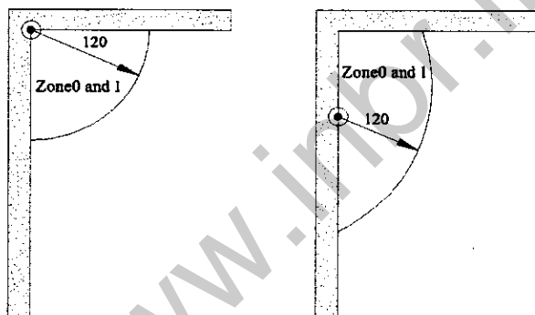
شکل ۱۳-۱۰-۴-۲: طرحواره موقعیت و ابعاد مناطق (zone)ها در حمام بدون زیردوشی
