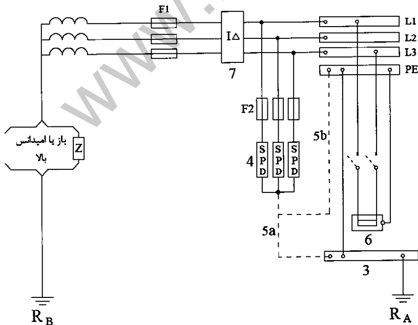
شکل ۴-۱۳-۱-۱۶-۳:۴ طرحواره نصب برقگیر حفاظتی در شبکه توزیع سیستم نیروی IT
