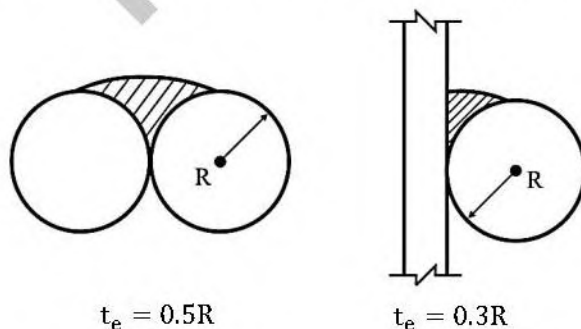
شکل ۱۰-۹-۲-۸: ضخامت مؤثر جوش‌های شیاری لب‌گرد
