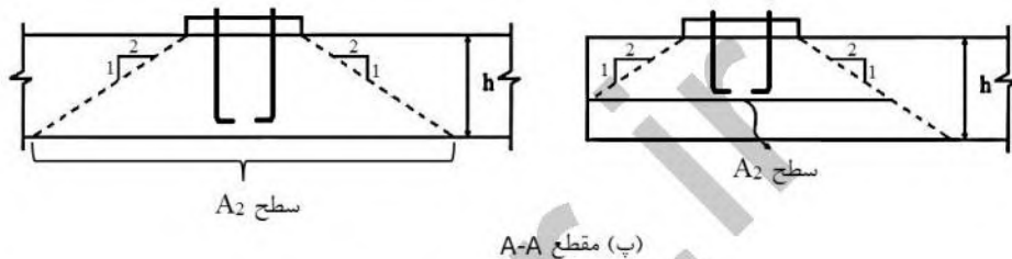
شکل ۲-۱۰-۹-۲۲: سطح اتکا در تماس با تکیه‌گاه بتنی
